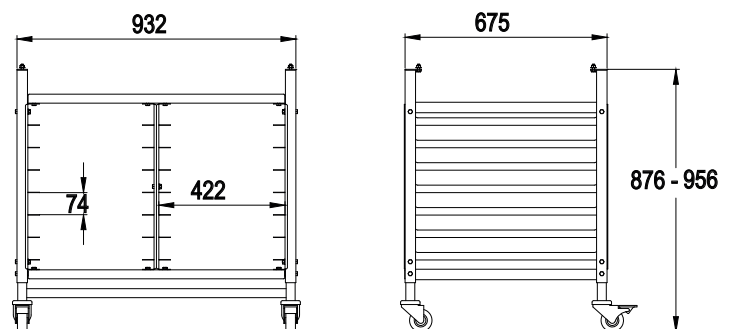
Dimensions inox avec rangement (en mm)
